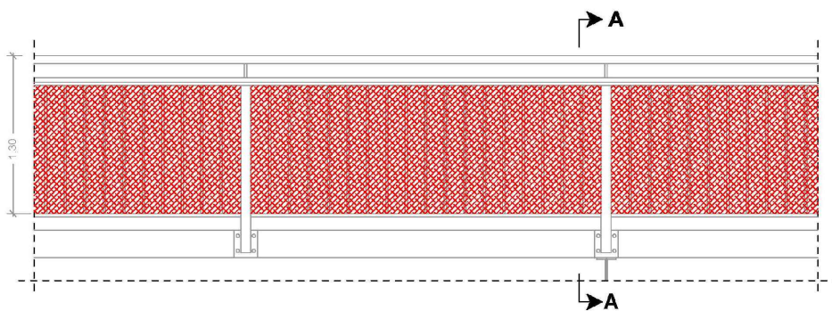
Draufsicht
