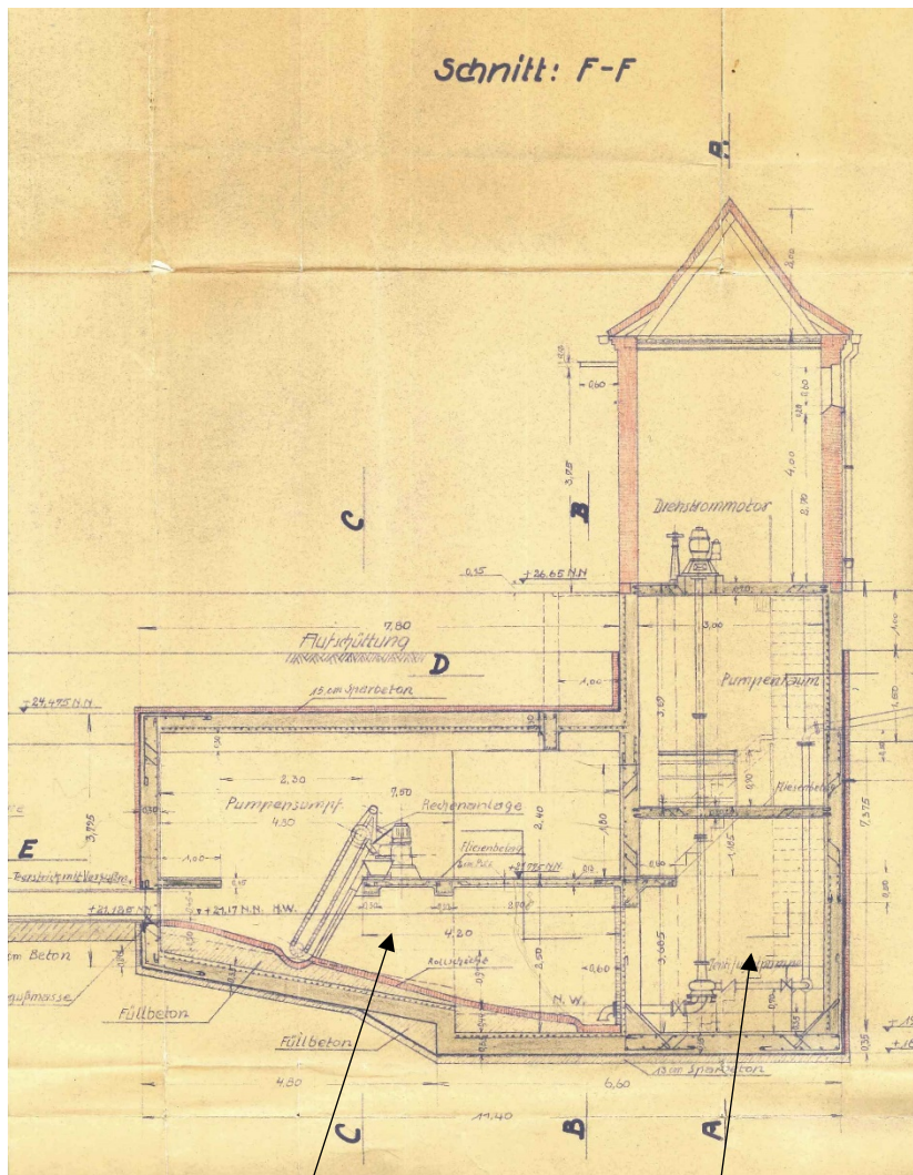
Vorkammer
