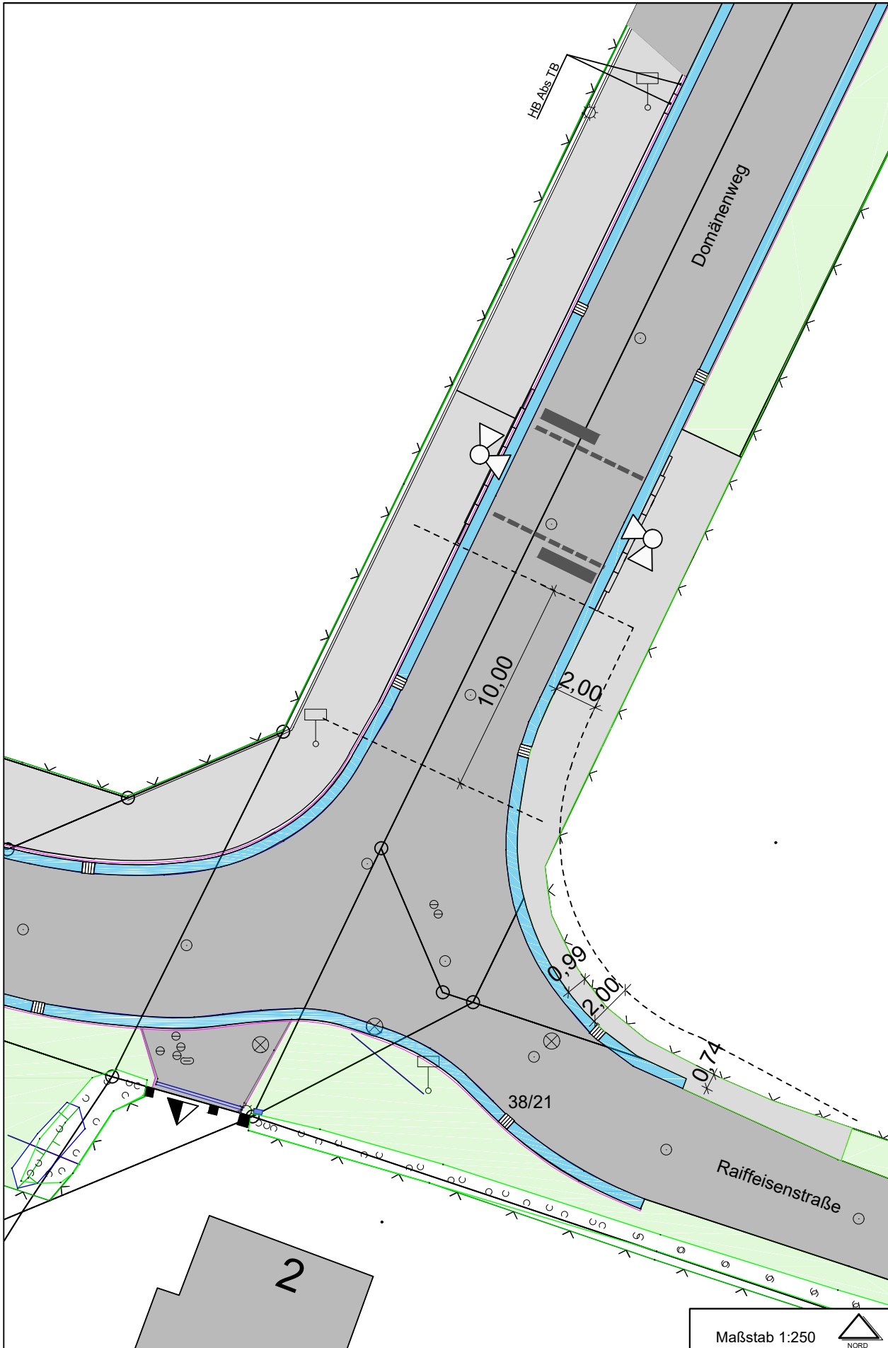
Herstellung des Fuß- und Radweges Domänenweg zwischen Südring und Raiffeisenstraße Variante 2: - Lichtsignalanlage -
