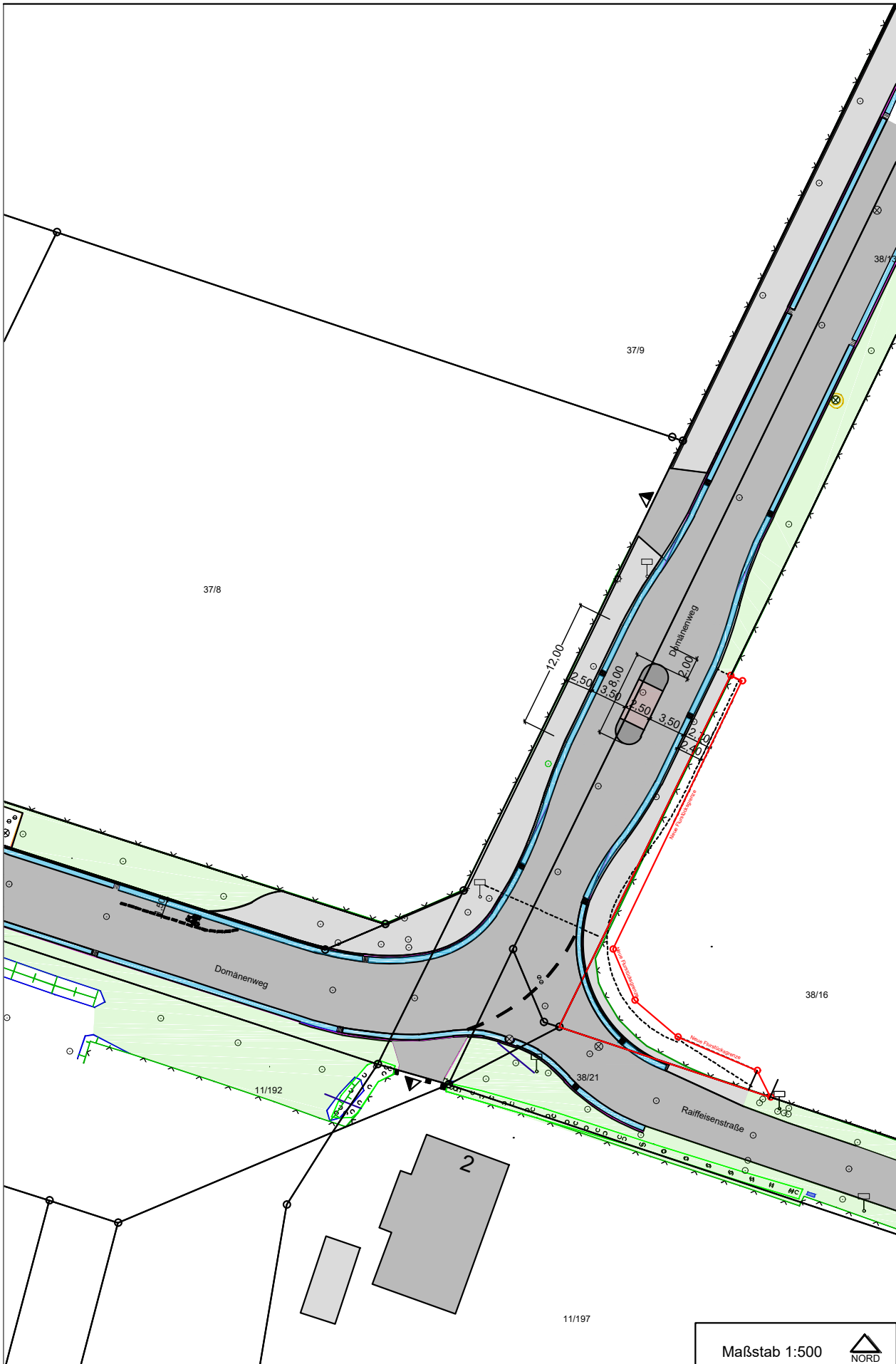
Herstellung des Fuß- und Radweges Domänenweg zwischen Südring und Raiffeisenstraße Variante 4: - Querungshilfe -
